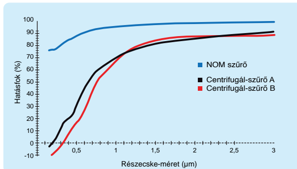
A NOM főszűrőjének hatásfoka, tipikus centrifugál-szűrőkkel összehasonlítva, DOP-pal mérve.
