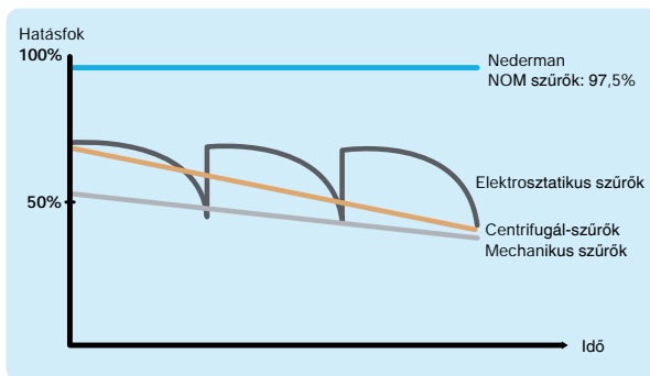
Különbőle olajkód-szűrők teljesítménye HEPA-szűrő nélkül Részecske-méret: <10 micron
